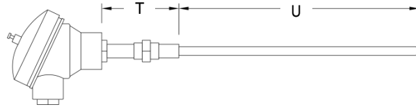
NEMA 4X CONEXIÓN NPT T/U 6" LONG. STD.
